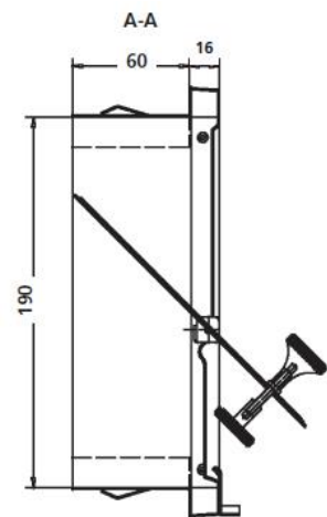
Regelklappe geöffnet dargestellt
